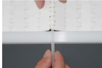
Insert rod
