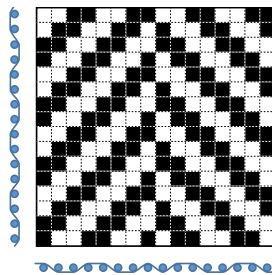
Armature en chevrons
